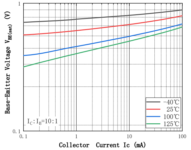
Fig. 4 - Base-Emmitter Voltage
